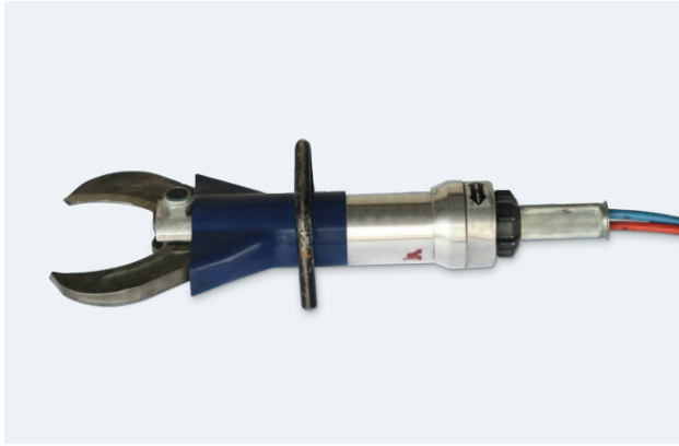
Hydraulische Schere
