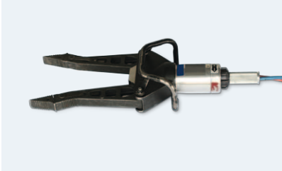
Hydraulischer Spreizer
