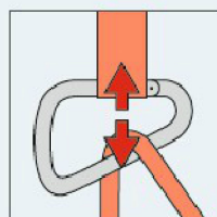
Querbelastung
