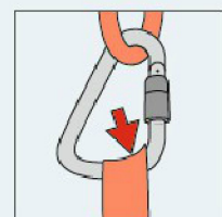
Momenteinwirkung
